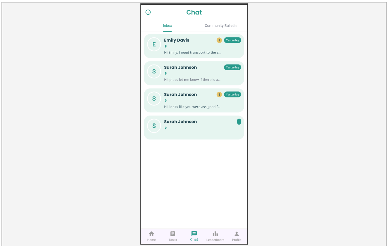
Chat inbox
